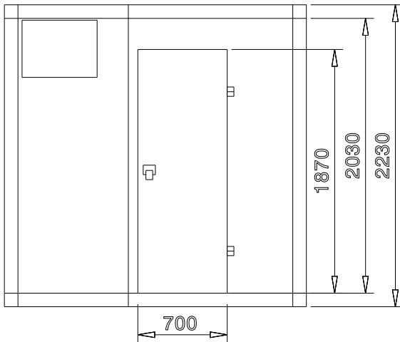
Zij aanzicht
